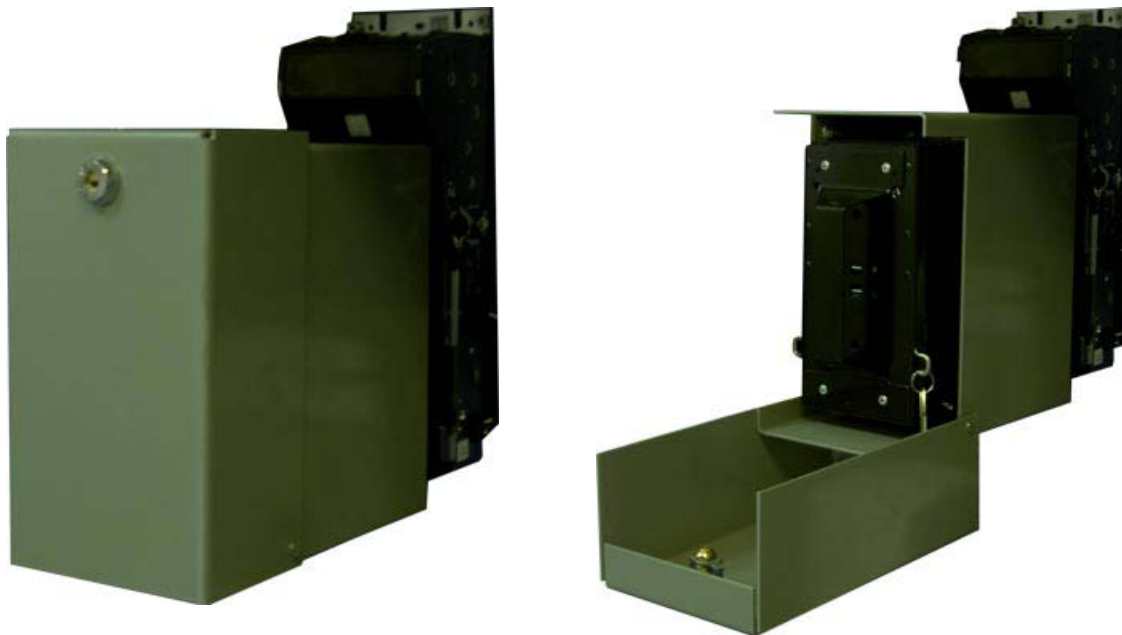
Рис. 16. Инкассация купюроприемника
