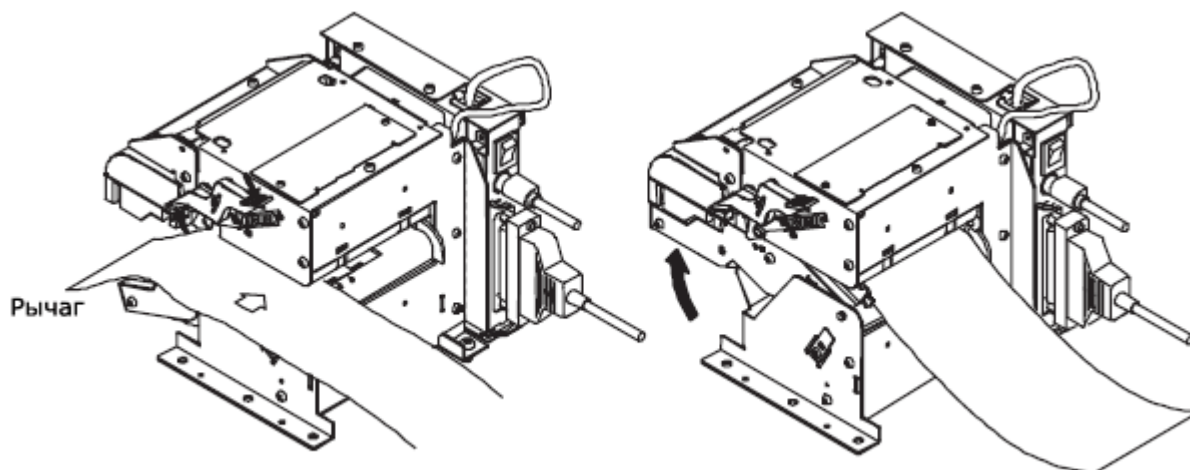
Рис. 28. Ручная замена термобумаги
