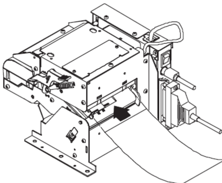
Рис. 29. Автоматическая замена термобумаги
