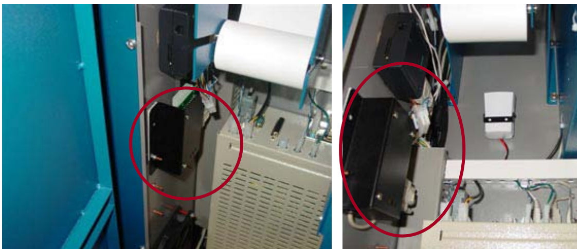
Рис. 11. Сторожевой таймер
