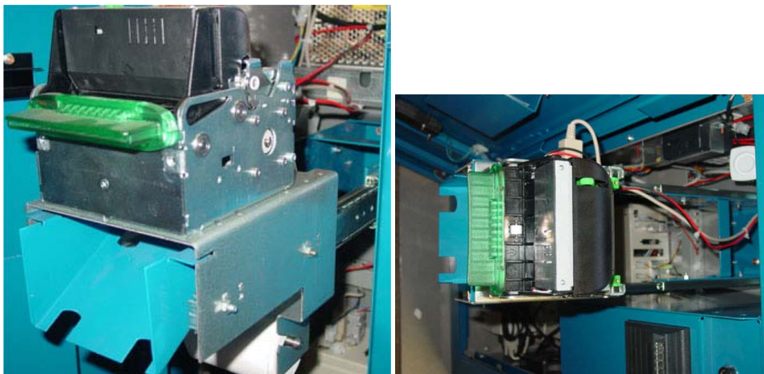
Рис. 27. Установка принтера Citizen PPU-700 на «салазках»
