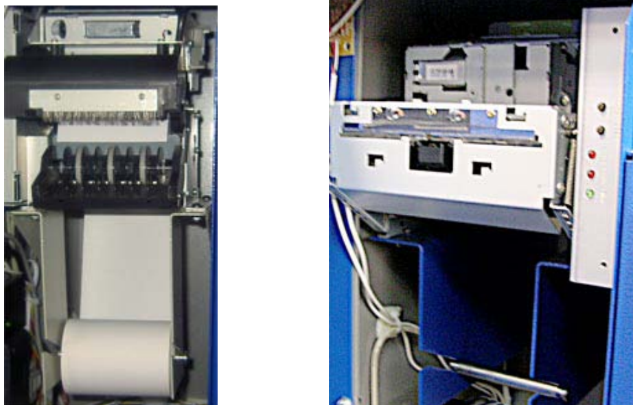
Рис. 6. Принтер
