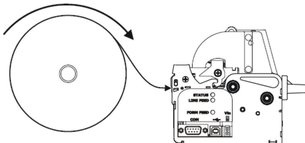
Рис. 32. Замена термобумаги
