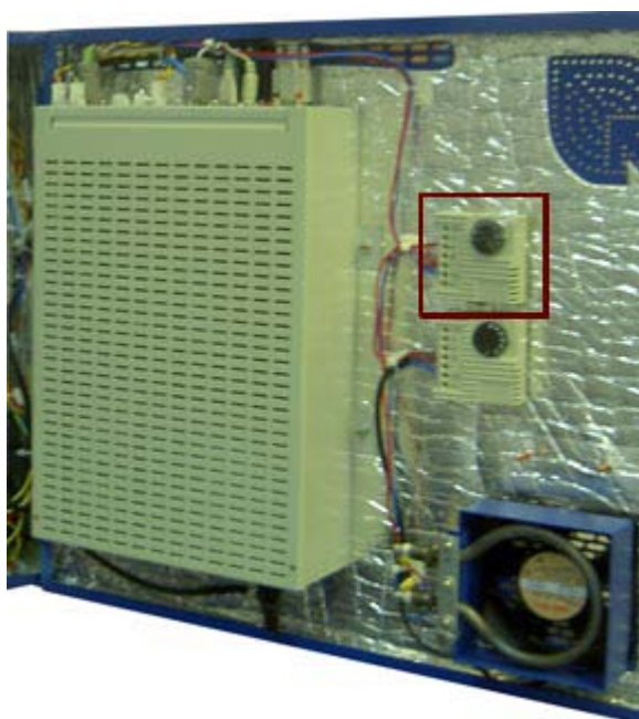
Рис. 14. Датчик включения вентилятора
