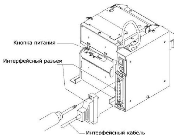
Рис. 17. Замена термобумаги
